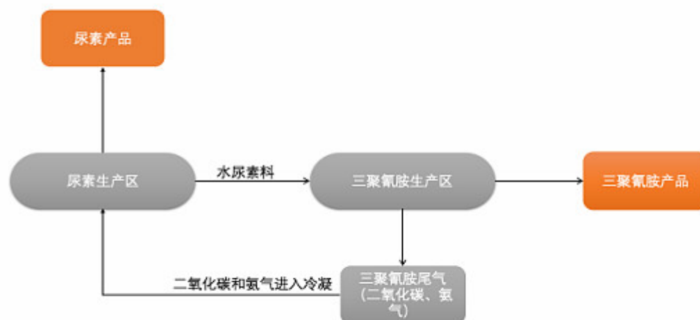
图 23：三聚氰胺尿素联合生产示意简图
